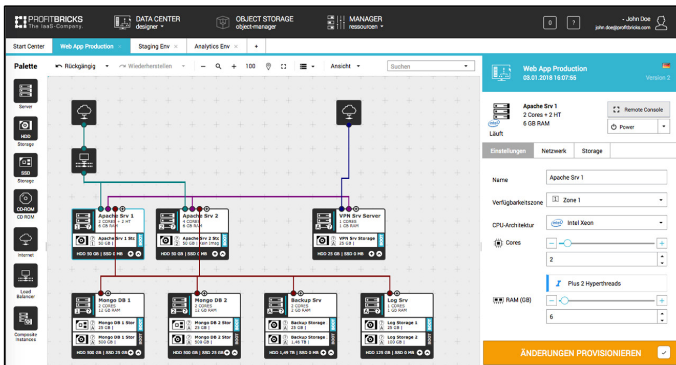
Abbildung 2: Grafische Oberfläche des Data Center Designers von ProfitBricks
